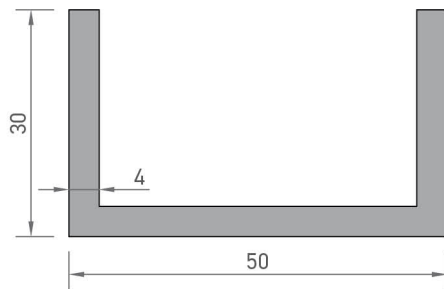
8454 U PROFİLİ 1,106 kg/mt
