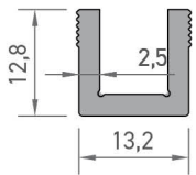
3902 U PROFİLİ 0,234 kg/mt
