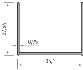
7615 U PROFİLİ 0,224 kg/mt
