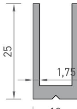
2141 U PROFİLİ 0,314 kg/mt
