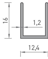
2222 U PROFİLİ 0,136 kg/mt
