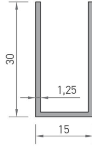
3889 U PROFİLİ 0,246 kg/mt
