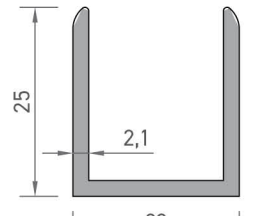
6861 U PROFİLİ 0,380 kg/mt
