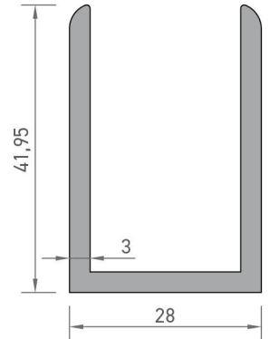
6859 U PROFİLİ 0,848 kg/mt
