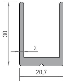
4255 U PROFİLİ 0,500 kg/mt
