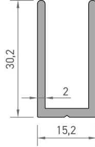
2154-A U PROFİLİ 0,394 kg/mt
