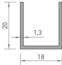
7550 U PROFİLİ 0,195 kg/mt
