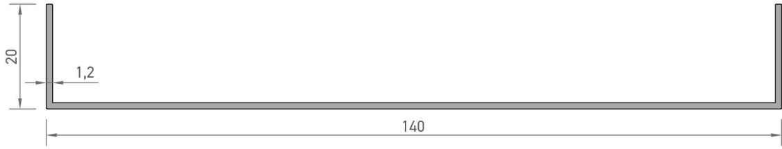
5430 U PROFİLİ 0,578 kg/mt
