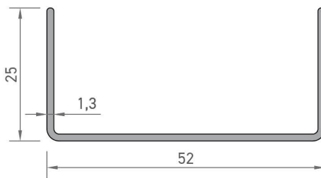
7954 U PROFİLİ 0,344 kg/mt
