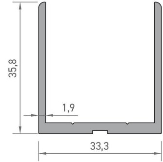
2251 U PROFİLİ 0,595 kg/mt
