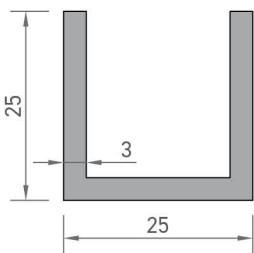
8491 U PROFİLİ 0,561 kg/mt
