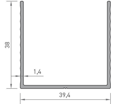
8024 U PROFİLİ 0,410 kg/mt
