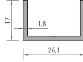
6226 U PROFİLİ 0,275 kg/mt
