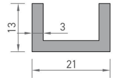
7042 U PROFİLİ 0,333 kg/mt
