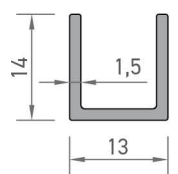
2223 U PROFİLİ 0,155 kg/mt
