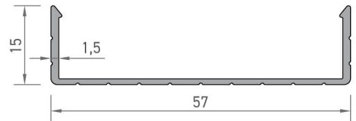
7592 U PROFİLİ 0,276 kg/mt
