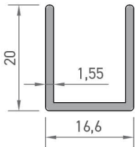
6896 U PROFİLİ 0,223 kg/mt
