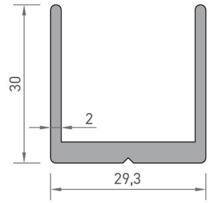
2534 GENİŞ U BAĞLANTI PROFİLİ 0,594 kg/mt
