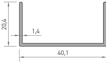
3624 U PROFİLİ 0,295 kg/mt
