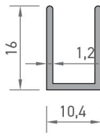
6079 U PROFİLİ 0,130 kg/mt
