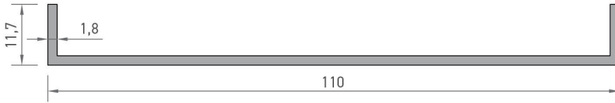
2825 U PROFİLİ 0,634 kg/mt
