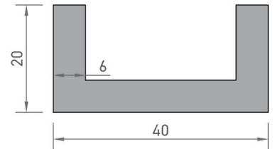
7699 U PROFİLİ 0,276 kg/mt
