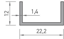
4595 U PROFİLİ 0,166 kg/mt
