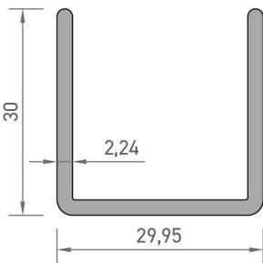
4709 U PROFİLİ 0,514 kg/mt
