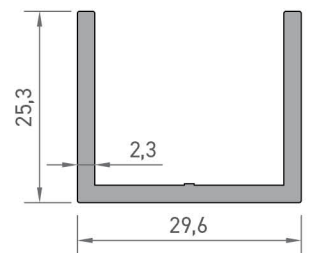
6564 U PROFİLİ 0,472 kg/mt
