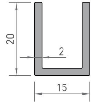
6918 U PROFİLİ 0,276 kg/mt
