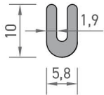
2242 U PROFİLİ 0,109 kg/mt
