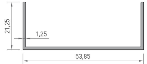
4643 U PROFİLİ 0,320 kg/mt
