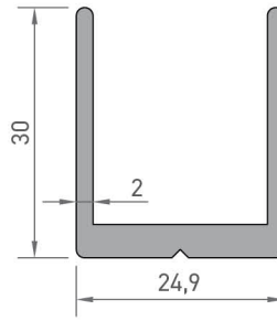
2814 U PROFİLİ 0,546 kg/mt
