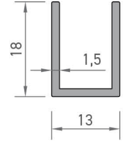
7915 U PROFİLİ 0,187 kg/mt
