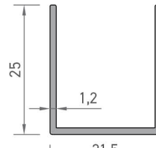
4515 U PROFİLİ 0,230 kg/mt
