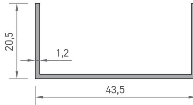
2747 U PROFİLİ 0,267 kg/mt
