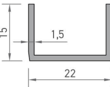
6213 U PROFİLİ 0,199 kg/mt
