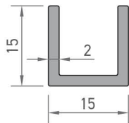
6914 U PROFİLİ 0,222 kg/mt
