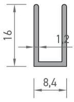
3327 U PROFİLİ 0,123 kg/mt
