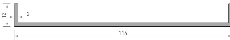
4896 U PROFİLİ 0,726 kg/mt
