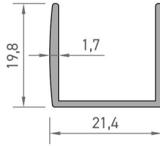
3415 U PROFİLİ 0,193 kg/mt
