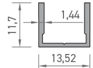
6795 U PROFİLİ 0,114 kg/mt
