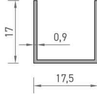
2221 U PROFİLİ 0,122 kg/mt
