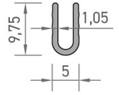
3335 U PROFİLİ 0,059 kg/mt
