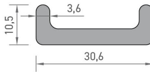
7442 U PROFİLİ 0,464 kg/mt
