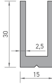
2154 U PROFİLİ 0,540 kg/mt
