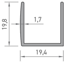
3446 U PROFİLİ 0,199 kg/mt
