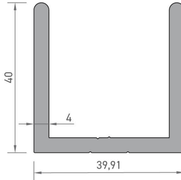
4922 U PROFİLİ 1,204 kg/mt
