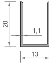
7904 U PROFİLİ 0,150 kg/mt
