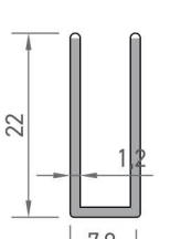
7790 U PROFİLİ 0,162 kg/mt
