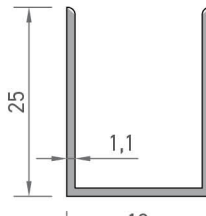
7903 U PROFİLİ 0,198 kg/mt
