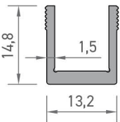
3903 U PROFİLİ 0,192 kg/mt
