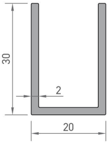
6917 U PROFİLİ 0,412 kg/mt
