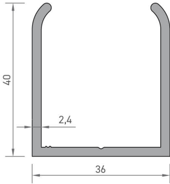
6646 U PROFİLİ 0,730 kg/mt
