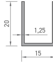
3888 U PROFİLİ 0,178 kg/mt
