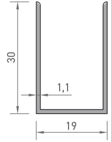
7905 U PROFİLİ 0,228 kg/mt
