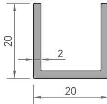
6915 U PROFİLİ 0,304 kg/mt
