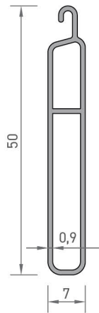
7623 ALT PARÇA PROFİLİ 0,265 kg/mt
