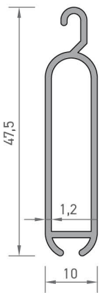
2217 FİTİLLİ ALT PARÇA PROFİLİ 0,340 kg/mt
