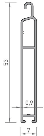
9113 ALT ETEK PROFİLİ 0,293 kg/mt
