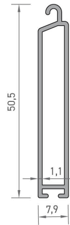
2849 ALT ETEK PROFİLİ 0,336 kg/mt
