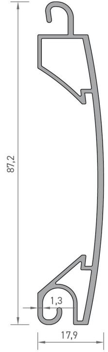
6144 PALET PROFİLİ 0,675 kg/mt
