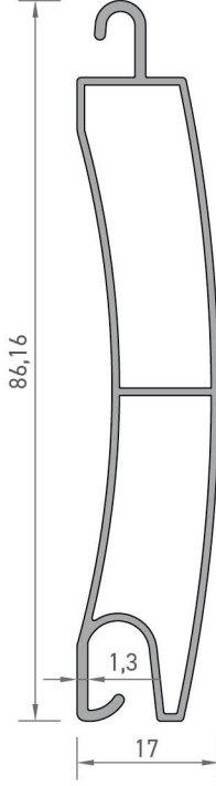
2978 PALET PROFİLİ 0,564 kg/mt
