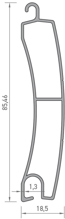
3060 PALET PROFİLİ 0,631 kg/mt
