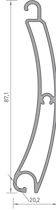
7401 PALET PROFİLİ 0,744 kg/mt
