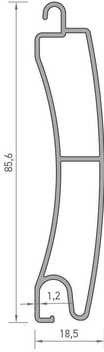
2213 PALET PROFİLİ 0,704 kg/mt
