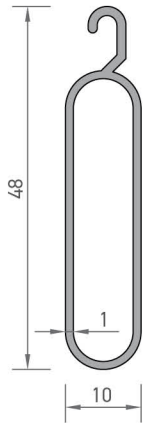
2218 ALT PARÇA PROFİLİ 0,295 kg/mt
