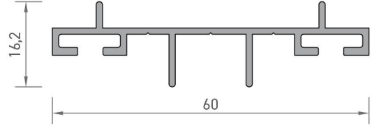
2268 IŞIKLI ALT PROFİLİ 0,400 kg/mt
