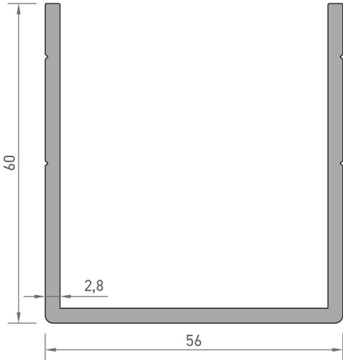
3451 KOMPOZİT "U" PROFİLİ 1,290 kg/mt
