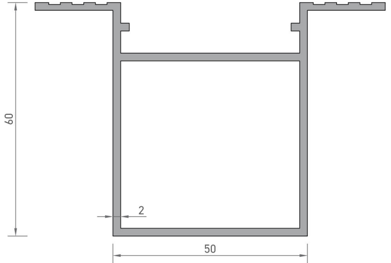
3452 KOMPOZİT KASA PROFİLİ 1,365 kg/mt
