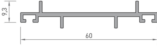
4904 IŞIKLI ALT PROFİLİ 0,390 kg/mt
