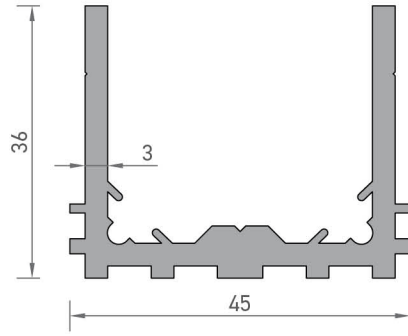
3493 KOMPOZİT BAĞLANTI PROFİLİ 1,055 kg/mt
