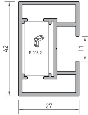
8166 KANAT PROFİLİ 0,723 kg/mt
