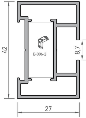
6798 KANAT PROFİLİ 0,677 kg/mt
