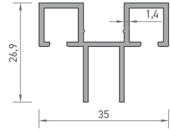
3919 JALUZİ KAPAK PROFİLİ 0,421 kg/mt
