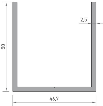
4152 U PROFİLİ 0,395 kg/mt
