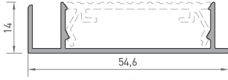
9024 SÜPÜRGELİK PROFİLİ 0,322 kg/mt
