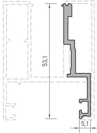
9035 KASA PROFİLİ 0,369 kg/mt
