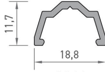
4146 KAPAK PROFİLİ 0,150 kg/mt
