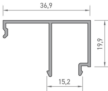
5598 CAM ÇİTASI PROFİLİ 0,315 kg/mt
