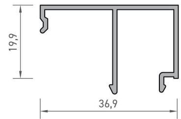
5598 ÇİTA PROFİLİ 0,315 kg/mt
