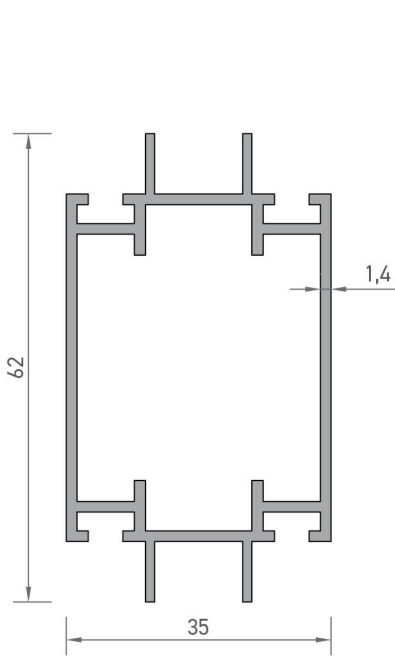
3920 JALUZİ KASA PROFİLİ 0,851 kg/mt
