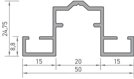
4145 KAPAK ALTI PROFİLİ 0,510 kg/mt
