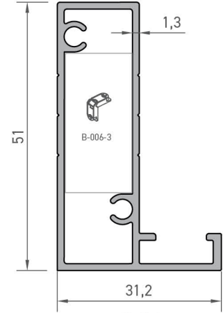
6796 KASA PROFİLİ 0,600 kg/mt
