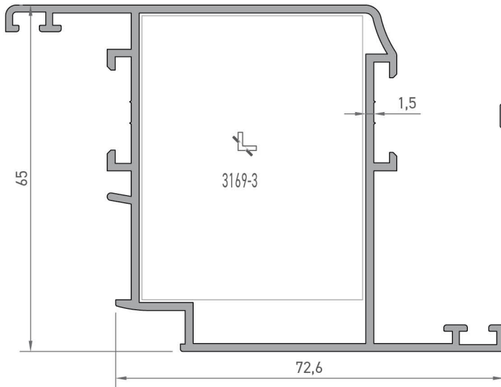
2585 KANAT PROFİLİ 1,275 kg/mt
