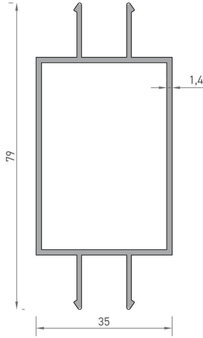
2451 JALUZİ KASA PROFİLİ 0,820 kg/mt
