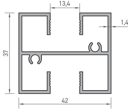
9056 KASA PROFİLİ 0,800 kg/mt
