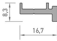
4150 SABİTLEME TAKOZ PROFİLİ 0,145 kg/mt
