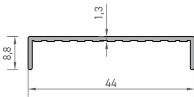
6143 ÇİTA PROFİLİ 0,188 kg/mt
