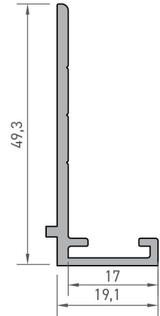
9057 KANAT ADAPTÖR PROFİLİ 0,400 kg/mt
