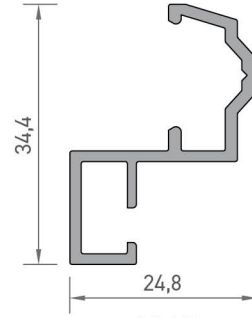
4147 KAPAK ALTI PROFİLİ 0,300 kg/mt
