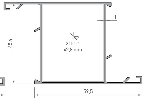
2181 GENİŞ KANAT PROFİLİ 0,645 kg/mt
