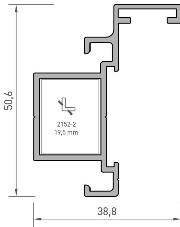
8779 KANAT ADAPTÖR PROFİLİ 0,613 kg/mt
