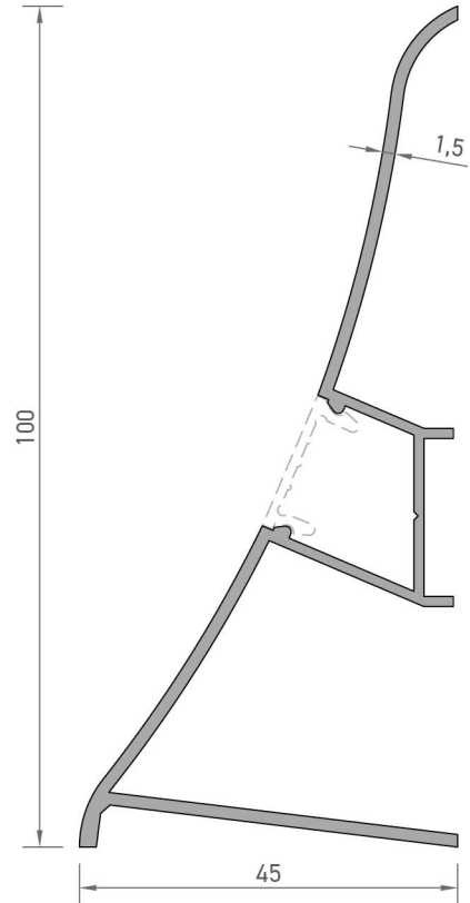
4653 SÜPÜRGELİK PROFİLİ 0,761 kg/mt
