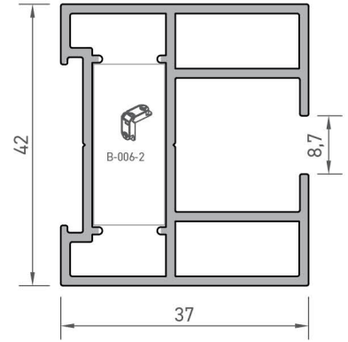
8811 KANAT PROFİLİ 0,877 kg/mt
