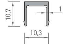
4491 DİKME KAPAK PROFİLİ 0,99 kg/mt
