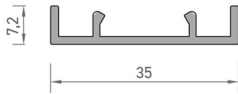
2452 JALUZİ KAPAK PROFİLİ 0,227 kg/mt
