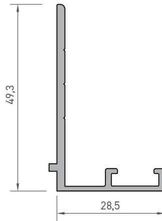
6961 KANAT ADAPTÖR PROFİLİ 0,428 kg/mt
