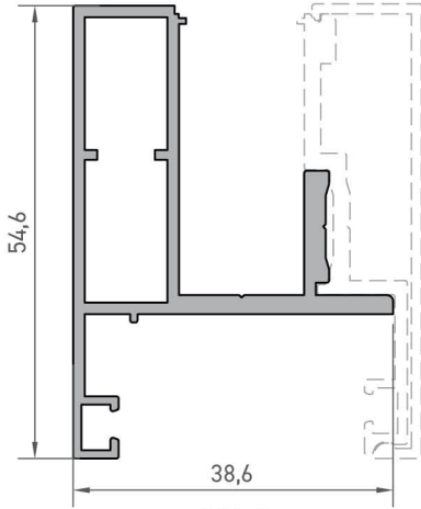
9034 KASA PROFİLİ 0,724 kg/mt
