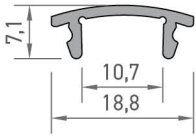
4149 KAPAK PROFİLİ 0,110 kg/mt
