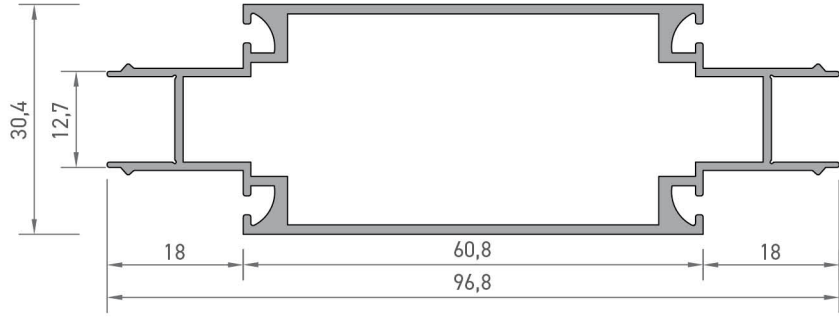
911 DİKME PROFİLİ 0,946 kg/mt
