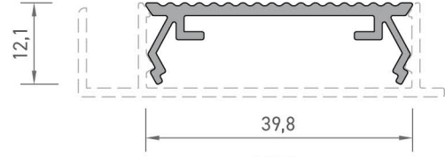
9025 SÜPÜRGELİK PROFİLİ 0,290 kg/mt
