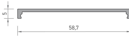
4949 DİKME KAPAK PROFİLİ 0,277 kg/mt
