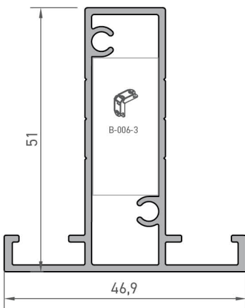
6797 ORTA KAYIT PROFİLİ 0,694 kg/mt
