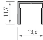
6795 ÇİTA PROFİLİ 0,114 kg/mt
