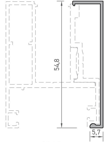
9036 KASA PROFİLİ 0,236 kg/mt
