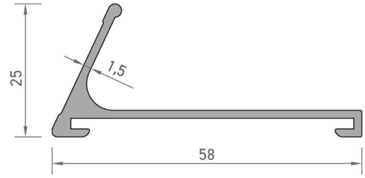
3453 MOBİLYA TUTAMAK PROFİLİ 0,434 kg/mt
