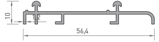
2879 KAYAR DOLAP PROFİLİ 0,315 kg/mt
