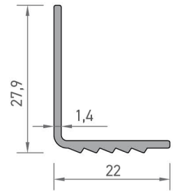
2256 DOLAP BAZA PROFİLİ 0,198 kg/mt
