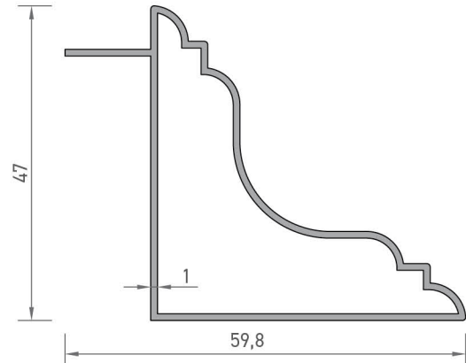
3124 MOBİLYA ÇERÇEVE PROFİLİ 0,494 kg/mt
