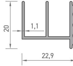
2255 DEKORATİF SÜRME CAM "E" PROFİLİ 0,241 kg/mt
