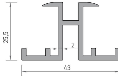
4611 RAF DUVAR PROFİLİ 0,610 kg/mt
