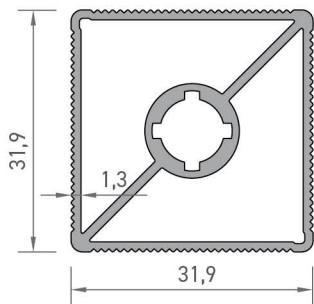
2709 32'LİK AYAK MOBİLYA PROFİLİ 0,628 kg/mt
