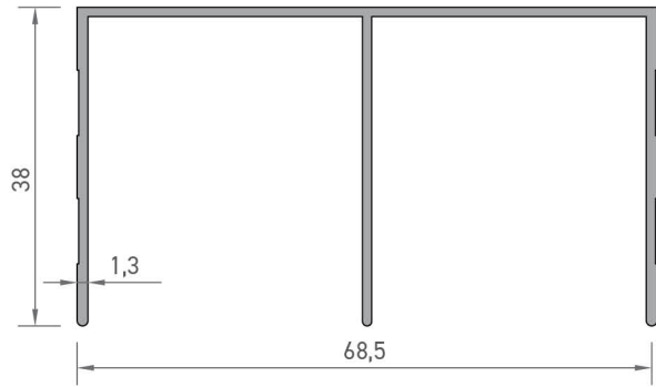
2874 KAYAR DOLAP PROFİLİ 0,558 kg/mt
