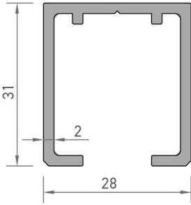
3207 ASKI RAY PROFİLİ 0,546 kg/mt
