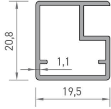
3423 MOBİLYA PROFİLİ 0,267 kg/mt
