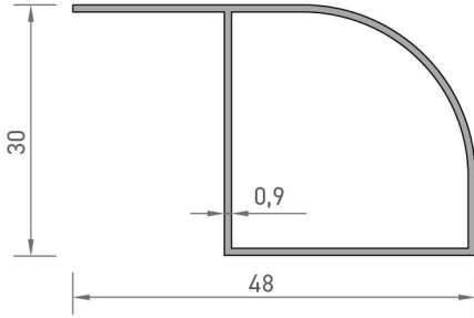
2253 KULAKLI KÖŞEYE DÖNÜŞ PROFİLİ 0,292 kg/mt
