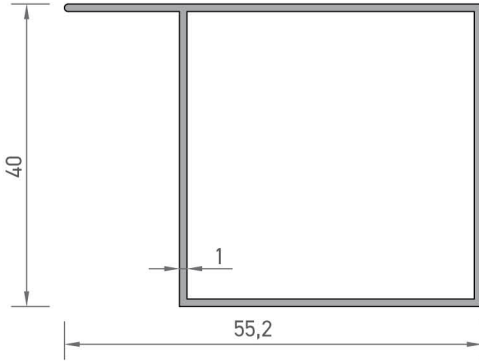
4214 KÖŞE DÖNÜŞ PROFİLİ 0,441 kg/mt
