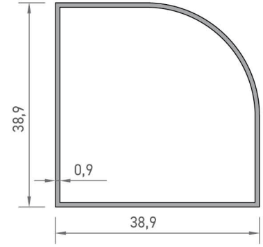
2252 KÖŞE DÖNÜŞ PROFİLİ 0,335 kg/mt
