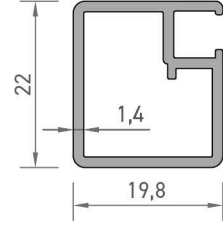
2907 MOBİLYA PROFİLİ 0,321 kg/mt
