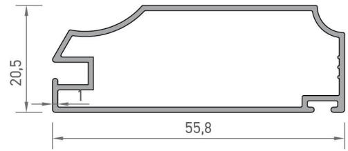
3123 MOBİLYA ÇERÇEVE PROFİLİ 0,437 kg/mt
