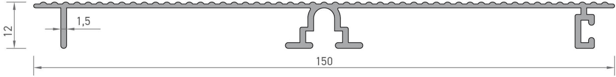
2719 DOLAP BAZA PROFİLİ 0,757 kg/mt
