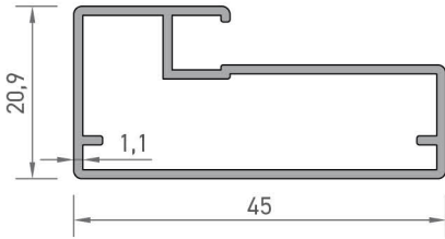
3287 MOBİLYA PROFİLİ 0,418 kg/mt
