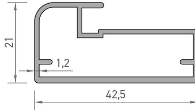
2844 MOBİLYA PROFİLİ 0,482 kg/mt
