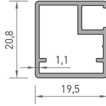
3412 MOBİLYA PROFİLİ 0,275 kg/mt
