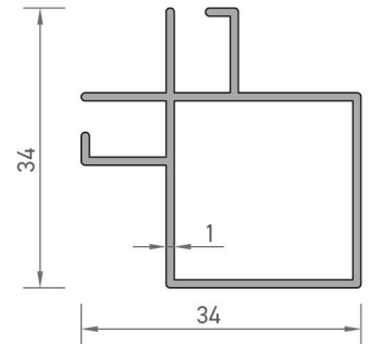
3126 MOBİLYA PROFİLİ 0,373 kg/mt
