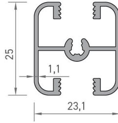
2880 KAYAR DOLAP PROFİLİ 0,366 kg/mt
