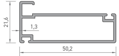
2947 MOBİLYA PROFİLİ 0,524 kg/mt
