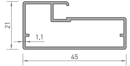
2945 MOBİLYA PROFİLİ 0,418 kg/mt
