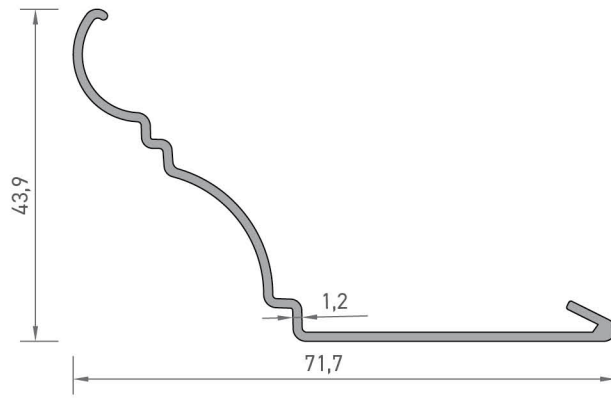
4215 MOBİLYA ÇERÇEVE PROFİLİ 0,361 kg/mt
