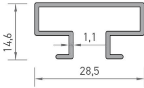
2905 MOBİLYA PROFİLİ 0,237 kg/mt
