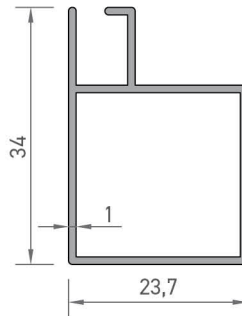
3125 MOBİLYA PROFİLİ 0,309 kg/mt
