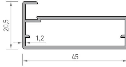
4864 MOBİLYA PROFİLİ 0,444 kg/mt
