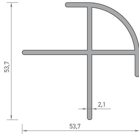
2906 KÖŞE DÖNÜŞ PROFİLİ 0,890 kg/mt
