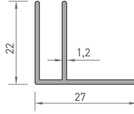
4514 MOBİLYA "F" PROFİLİ 0,225 kg/mt
