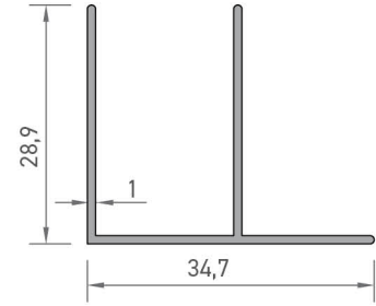
7630 MOBİLYA "F" PROFİLİ 0,245 kg/mt
