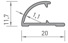
2716 HALI BİTİM PROFİLİ 0,125 kg/mt
