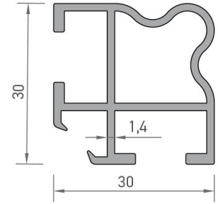
3450 KAYAR DOLAP PROFİLİ 0,553 kg/mt
