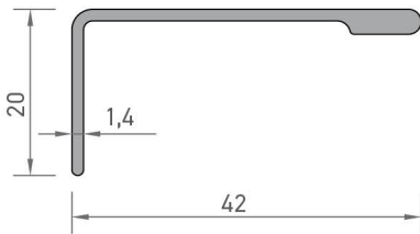
4943 MOBİLYA TUTAMAK PROFİLİ 0,265 kg/mt
