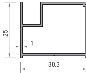
3049 MOBİLYA KAPAK PROFİLİ 0,315 kg/mt
