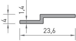
4508 MOBİLYA "Z" PROFİLİ 0,100 kg/mt
