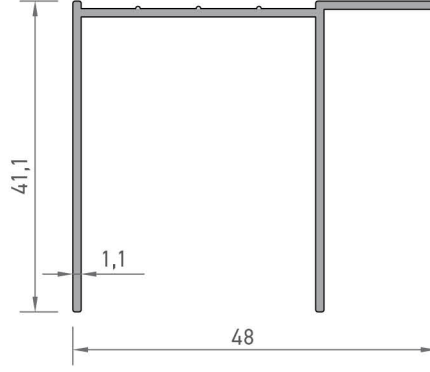
3050 MOBİLYA PROFİLİ 0,385 kg/mt
