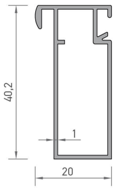
4213 MOBİLYA PROFİLİ 0,335 kg/mt
