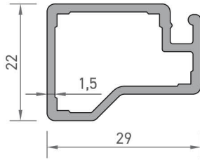
3238 MOBİLYA PROFİLİ 0,423 kg/mt
