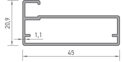
3286 MOBİLYA PROFİLİ 0,400 kg/mt
