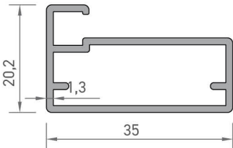
2099 MOBİLYA KAPAK PROFİLİ 0,395 kg/mt
