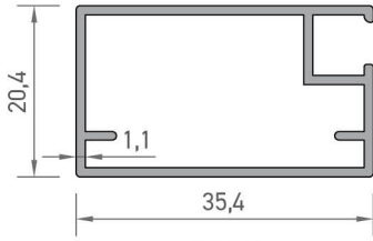
4412 MOBİLYA PROFİLİ 0,369 kg/mt
