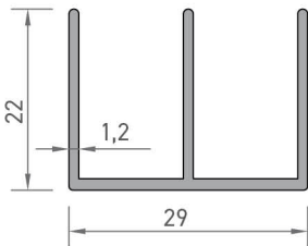
4513 MOBİLYA "E" PROFİLİ 0,312 kg/mt
