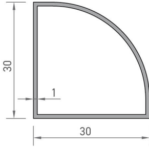
2254 KÖŞE DÖNÜŞ PROFİLİ 0,286 kg/mt
