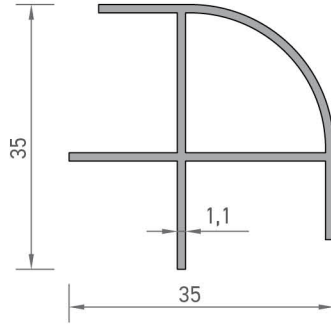
4402 KÖŞE DÖNÜŞ PROFİLİ 0,360 kg/mt
