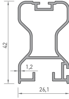
2877 KAYAR DOLAP PROFİLİ 0,540 kg/mt
