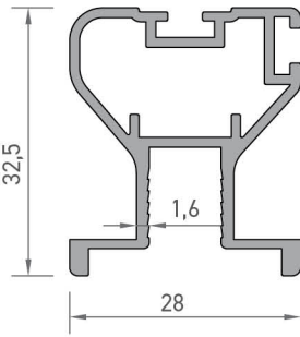
2878 KAYAR DOLAP PROFİLİ 0,506 kg/mt
