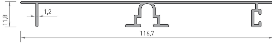
2720 DOLAP BAZA PROFİLİ 0,540 kg/mt
