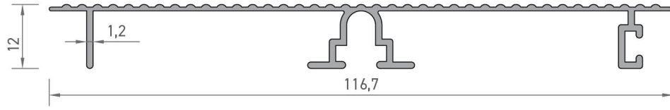
2718 DOLAP BAZA PROFİLİ 0,510 kg/mt
