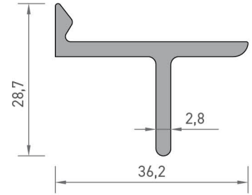
3069 MOBİLYA PROFİLİ 0,457 kg/mt
