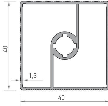
2710 40'LIK AYAK MOBİLYA PROFİLİ 0,730 kg/mt
