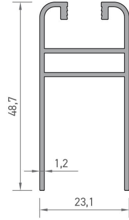
2876 KAYAR DOLAP PROFİLİ 0,505 kg/mt
