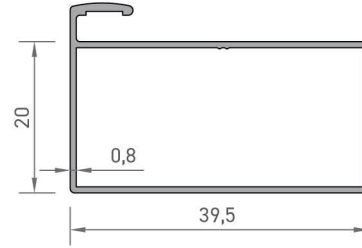
6636 SİNEKLİK MOBİLYA PROFİLİ 0,285 kg/mt
