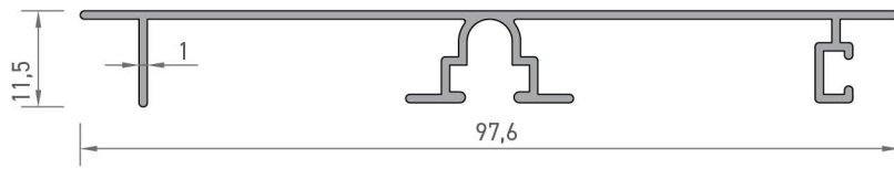
2721 DOLAP BAZA PROFİLİ 0,446 kg/mt
