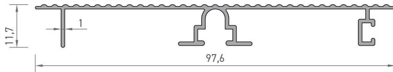
2717 DOLAP BAZA PROFİLİ 0,422 kg/mt
