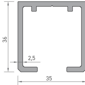
3209 ASKI RAY PROFİLİ 0,822 kg/mt
