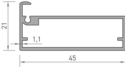
4484 MOBİLYA PROFİLİ 0,446 kg/mt
