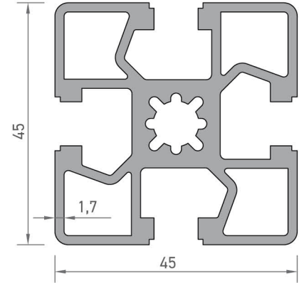
2711 45'LIK SİGMA PROFİLİ 1,820 kg/mt
