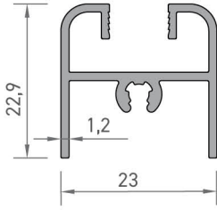
2875 KAYAR DOLAP PROFİLİ 0,320 kg/mt
