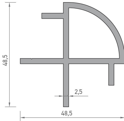
4660 KÖŞE DÖNÜŞ PROFİLİ 1,050 kg/mt
