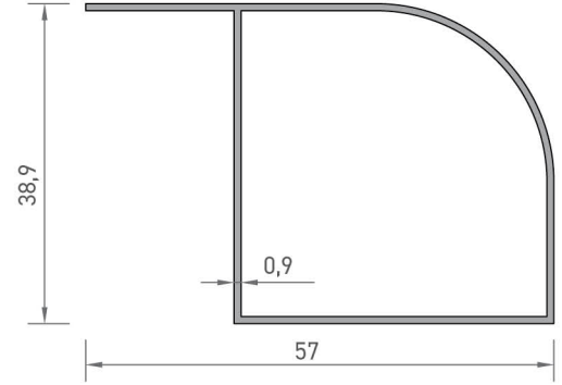
2248 KULAKLI KÖŞEYE DÖNÜŞ PROFİLİ 0,375 kg/mt
