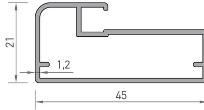
4413 MOBİLYA PROFİLİ 0,455 kg/mt
