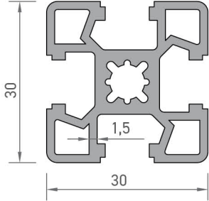
2712 30'LUK SİGMA PROFİLİ 0,880 kg/mt
