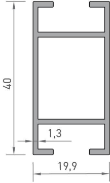
3454 KAYAR DOLAP PROFİLİ 0,470 kg/mt
