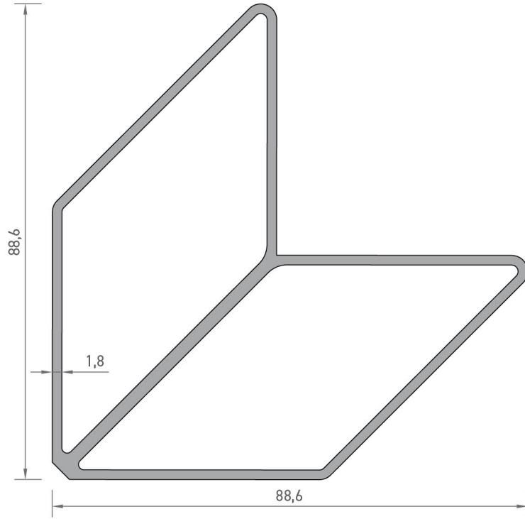
2421 KÖŞE BAĞLANTI PROFİLİ 1,820 kg/mt
