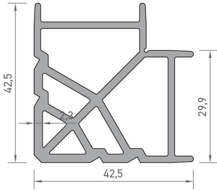
5274 DAR ÇAVUŞ KÖŞE BAĞLANTI PROFİLİ 7,348 kg/mt
