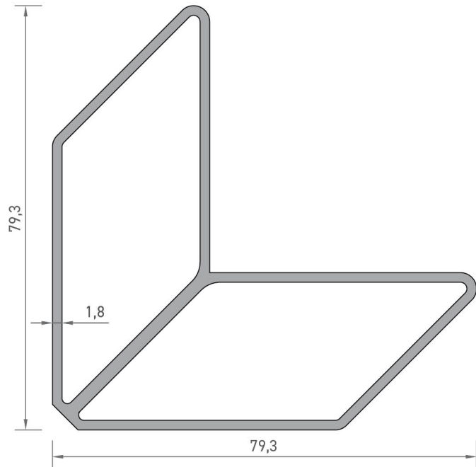
2400 KÖŞE BAĞLANTI PROFİLİ 1,577 kg/mt
