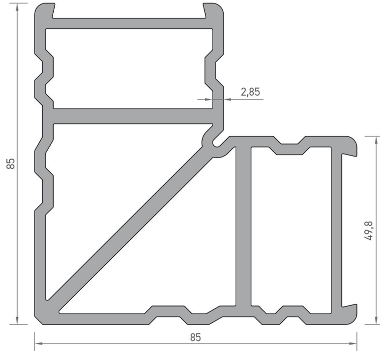
7154 KÖŞE BAĞLANTI TAKOZU PROFİLİ 4,293 kg/mt
