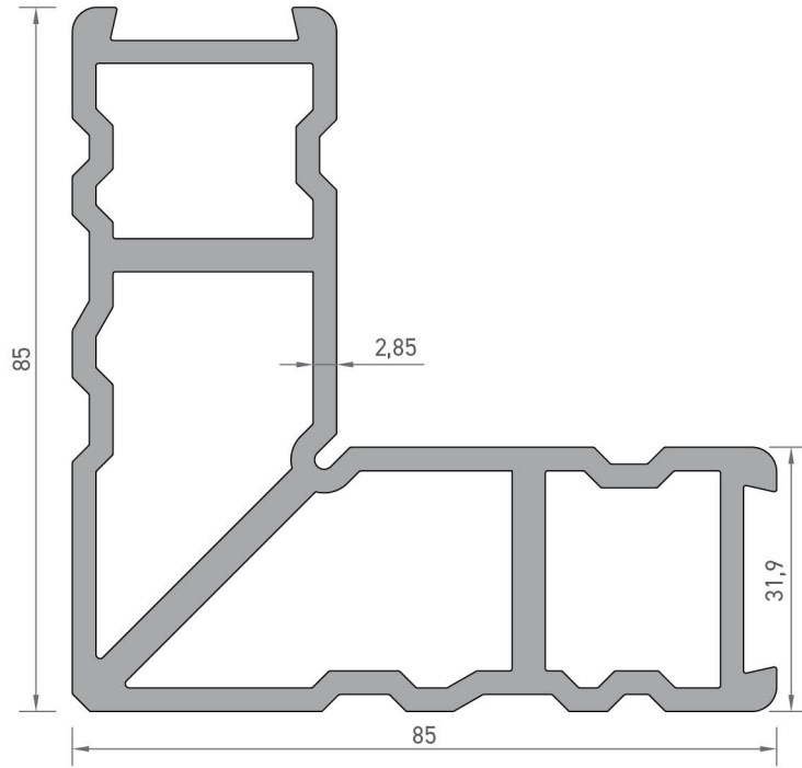
6936 KÖŞE BAĞLANTI TAKOZU PROFİLİ 3,640 kg/mt
