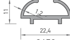
2450 PERDE RAY PROFİLİ 0,180 kg/mt
