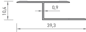
2087 HALI-SERAMİK BİRLEŞİM PROFİLİ 0,130 kg/mt
