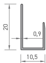
2093 HALI PROFİLİ 0,095 kg/mt
