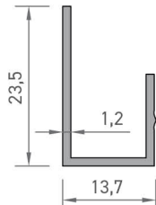
7245 HALI PROFİLİ 0,157 kg/mt
