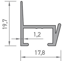
2247 PERDE RAY PROFİLİ 0,167 kg/mt
