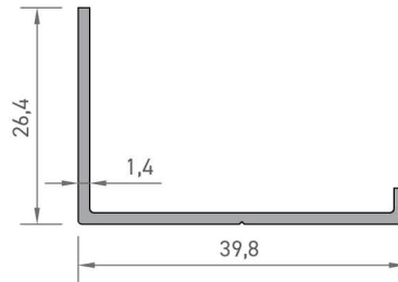
4474 HALI PROFİLİ 0,260 kg/mt
