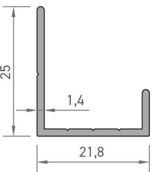
4783 HALI PROFİLİ 0,202 kg/mt
