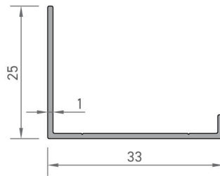
4895 HALI PROFİLİ 0,165 kg/mt
