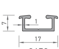
2453 PERDE RAY PROFİLİ 0,095 kg/mt
