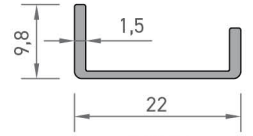
4955 HALI PROFİLİ 0,110 kg/mt
