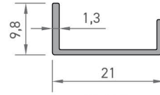
2761 HALI PROFİLİ 0,108 kg/mt
