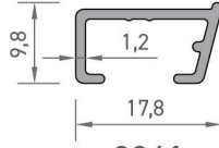
2241 PERDE RAY PROFİLİ 0,130 kg/mt
