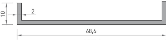
6854 U PROFİLİ 0,463 kg/mt
