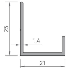
3488 HALI PROFİLİ 0,202 kg/mt
