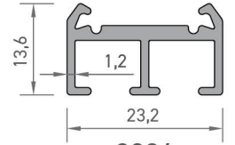
2886 PERDE RAY PROFİLİ 0,260 kg/mt
