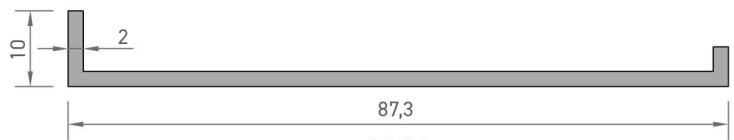
6846 HALI PROFİLİ 0,535 kg/mt
