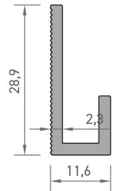
7444 HALI PROFİLİ 0,286 kg/mt
