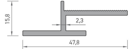
4929 HALI-SERAMİK BİRLEŞİM PROFİLİ 0,420 kg/mt
