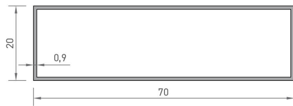
7306 KUTU PROFİLİ 0,430 kg/mt
