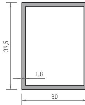
2408 KUTU PROFİLİ 0,648 kg/mt
