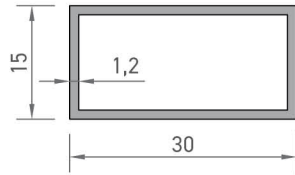
7425 KUTU PROFİLİ 0,276 kg/mt
