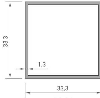
9246 KUTU PROFİLİ 0,440 kg/mt
