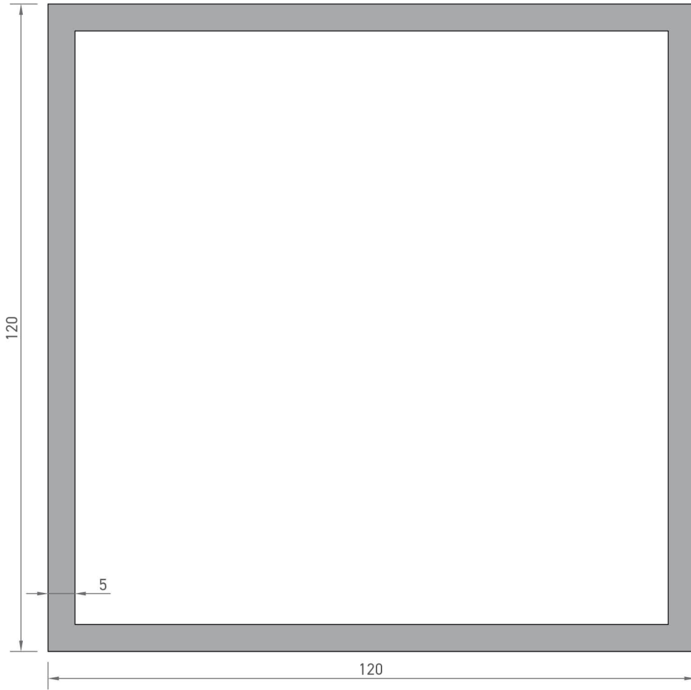
8452 KUTU PROFİLİ 6,233 kg/mt
