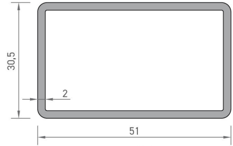
3237 KUTU PROFİLİ 0,827 kg/mt
