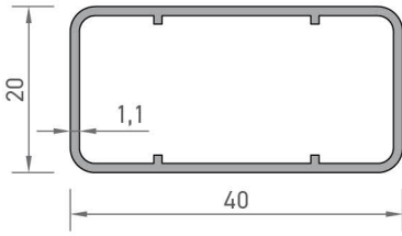
2988 KUTU PROFİLİ 0,343 kg/mt
