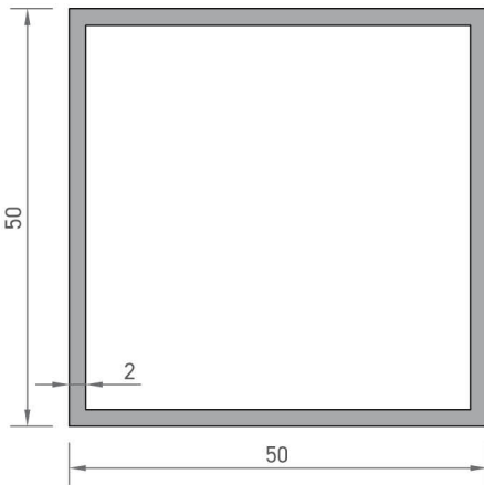
3836 KUTU PROFİLİ 1,041 kg/mt
