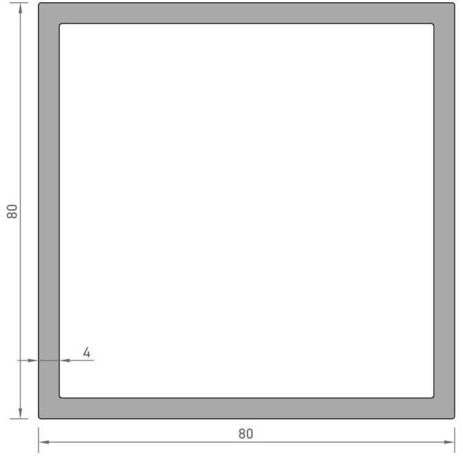
7648 KUTU PROFİLİ 3,295 kg/mt
