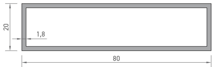
7328 KUTU PROFİLİ 1,015 kg/mt
