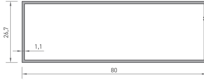
7876 KUTU PROFİLİ 0,623 kg/mt
