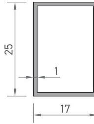
2167 KUTU PROFİLİ 0,217 kg/mt
