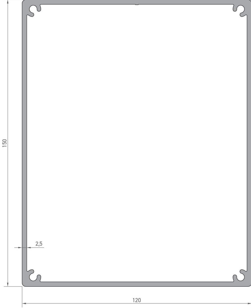
9254 KUTU PROFİLİ 3,755 kg/mt
