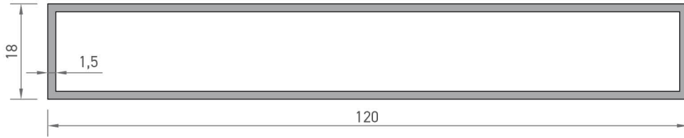
7665 KUTU PROFİLİ 1,097 kg/mt
