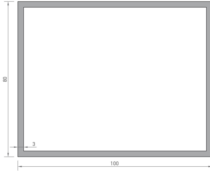
8543 KUTU PROFİLİ 2,829 kg/mt
