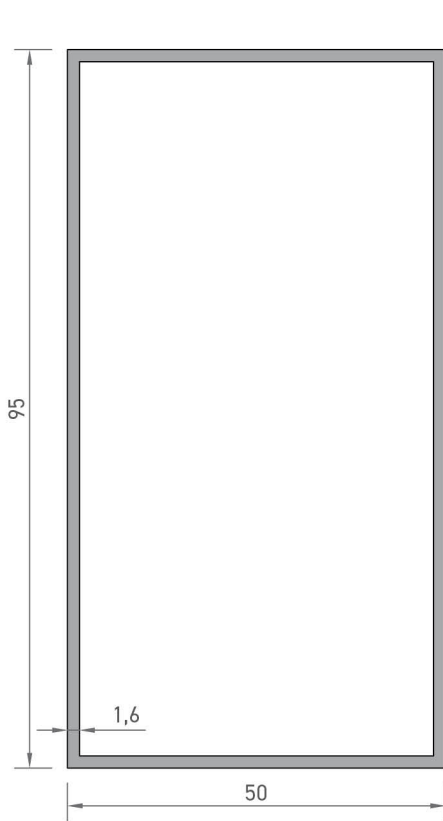
2169 KUTU PROFİLİ 1,230 kg/mt
