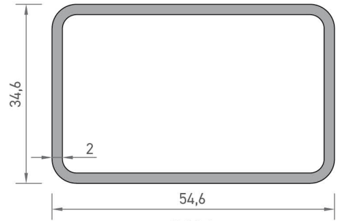
2991 KUTU PROFİLİ 0,886 kg/mt
