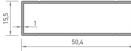
2409 KUTU PROFİLİ 0,344 kg/mt
