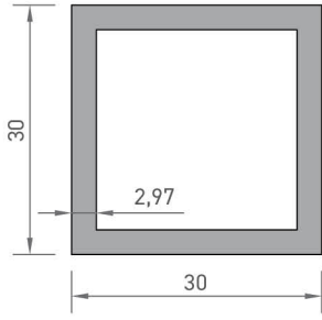
7818 KUTU PROFİLİ 0,878 kg/mt
