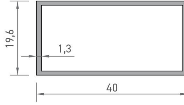
6126 KUTU PROFİLİ 0,362 kg/mt
