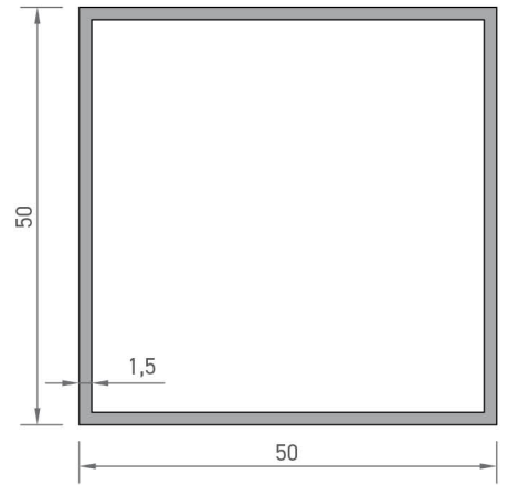
2873 KUTU PROFİLİ 0,789 kg/mt
