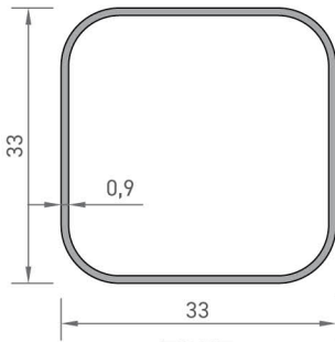
7305 KUTU PROFİLİ 0,303 kg/mt
