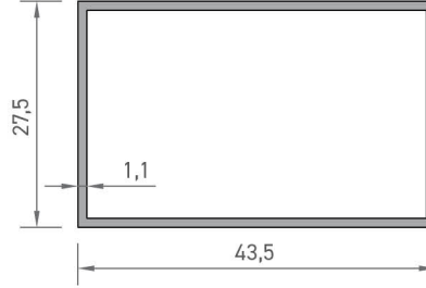
8930 KUTU PROFİLİ 0,410 kg/mt
