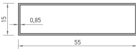
6278 KUTU PROFİLİ 0,315 kg/mt
