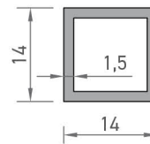
4239 KUTU PROFİLİ 0,204 kg/mt
