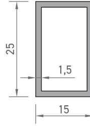
8324 KUTU PROFİLİ 0,301 kg/mt
