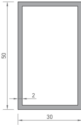
8323 KUTU PROFİLİ 0,825 kg/mt
