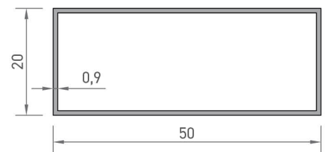
9198 KUTU PROFİLİ 0,315 kg/mt
