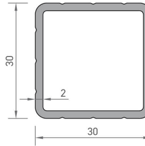
2798 KUTU PROFİLİ 0,582 kg/mt
