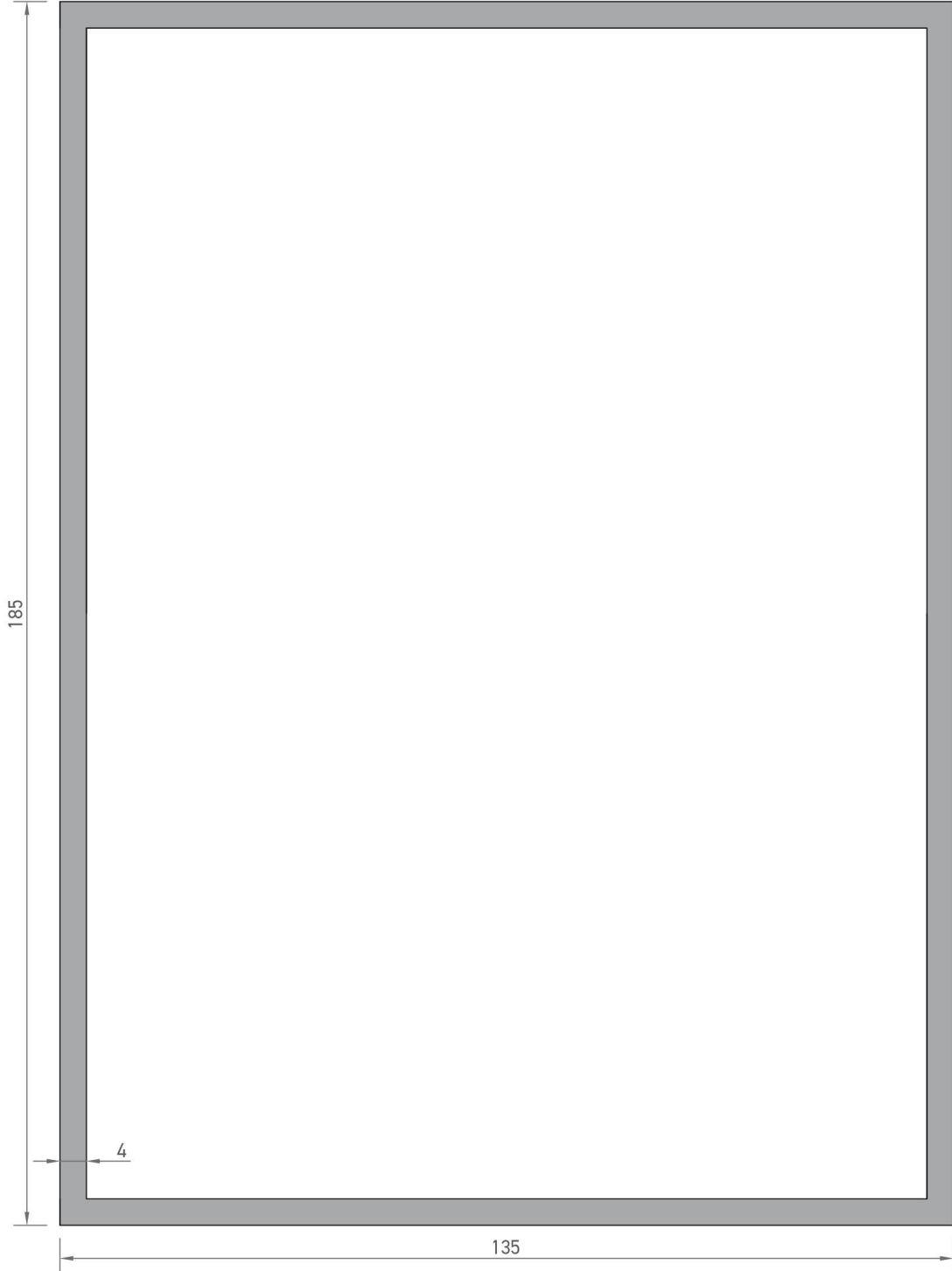
8702 KUTU PROFİLİ 6,765 kg/mt
