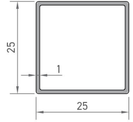
7922 KUTU PROFİLİ 0,260 kg/mt
