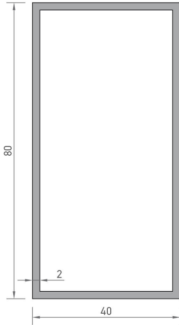
2257 KUTU PROFİLİ 1,258 kg/mt
