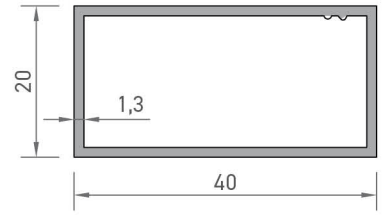
3399 KUTU PROFİLİ 0,407 kg/mt
