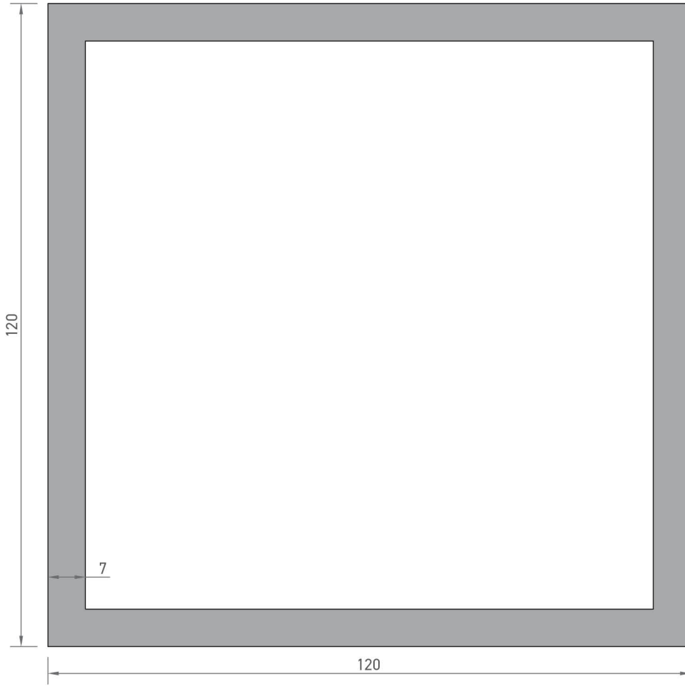
7059 KUTU PROFİLİ 8,575 kg/mt
