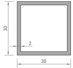
7723 KUTU PROFİLİ 0,607 kg/mt
