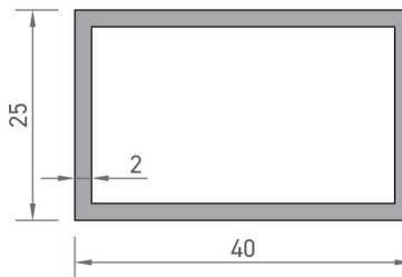
8745 KUTU PROFİLİ 0,661 kg/mt
