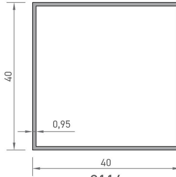
2116 KUTU PROFİLİ 0,403 kg/mt
