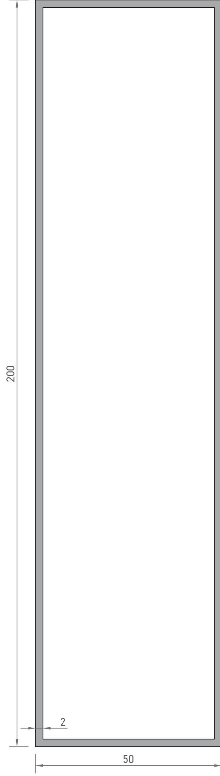
7559 KUTU PROFİLİ 2,657 kg/mt
