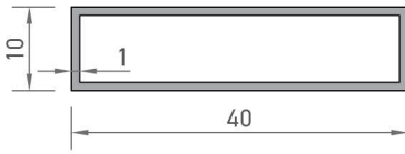
6774 KUTU PROFİLİ 0,260 kg/mt
