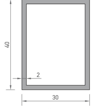
2396 KUTU PROFİLİ 0,721 kg/mt
