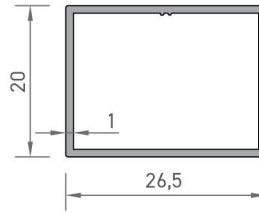
8211 KUTU PROFİLİ 0,250 kg/mt
