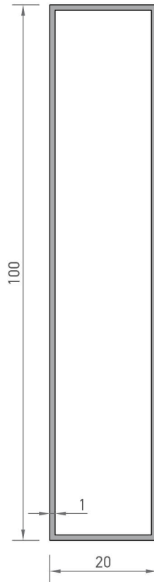
4841 KUTU PROFİLİ 0,640 kg/mt
