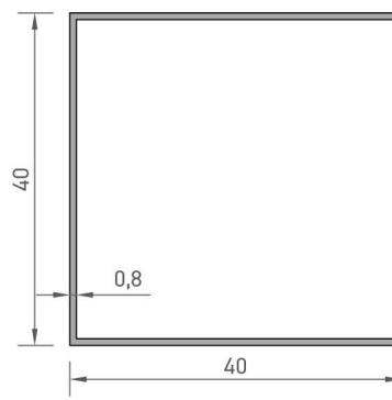
6427 KUTU PROFİLİ 0,339 kg/mt
