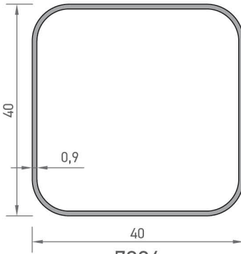
7304 KUTU PROFİLİ 0,355 kg/mt
