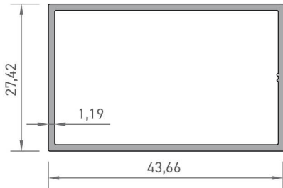
3708 KUTU PROFİLİ 0,444 kg/mt
