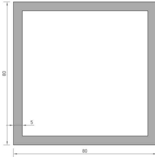
7057 KUTU PROFİLİ 4,065 kg/mt
