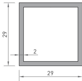
6678 KUTU PROFİLİ 0,585 kg/mt
