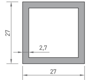
7819 KUTU PROFİLİ 0,715 kg/mt
