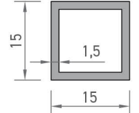
6919 KUTU PROFİLİ 0,220 kg/mt
