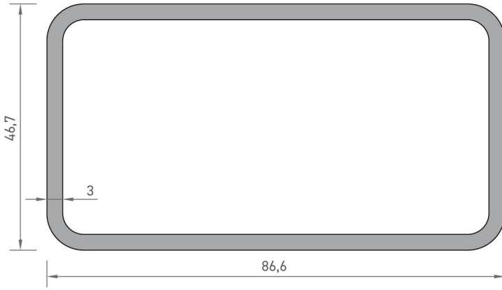
2993 KUTU PROFİLİ 1,994 kg/mt
