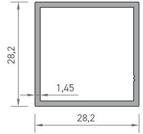
7877 KUTU PROFİLİ 0,420 kg/mt
