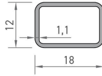
2984 KUTU PROFİLİ 0,153 kg/mt
