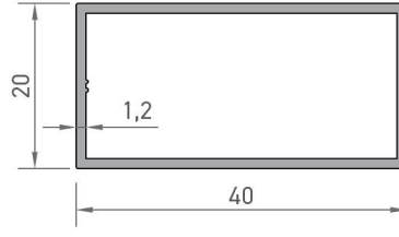
7857 KUTU PROFİLİ 0,375 kg/mt
