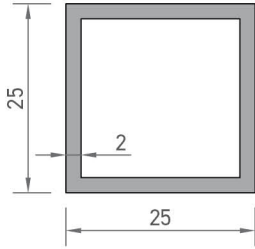
7722 KUTU PROFİLİ 0,499 kg/mt
