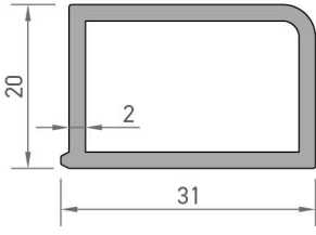
7491 KUTU PROFİLİ 0,494 kg/mt
