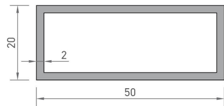
8415 KUTU PROFİLİ 0,715 kg/mt
