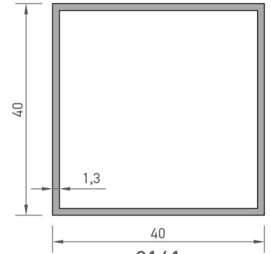
9141 KUTU PROFİLİ 0,544 kg/mt
