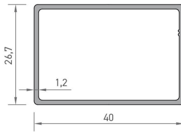
8530 KUTU PROFİLİ 0,420 kg/mt
