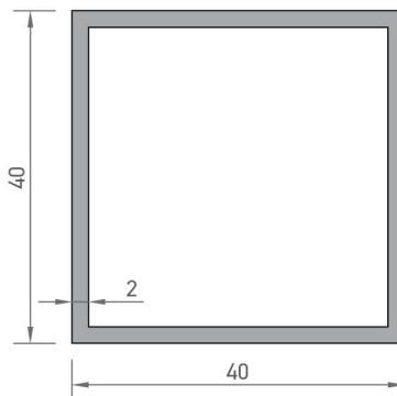
2209 KUTU PROFİLİ 0,825 kg/mt
