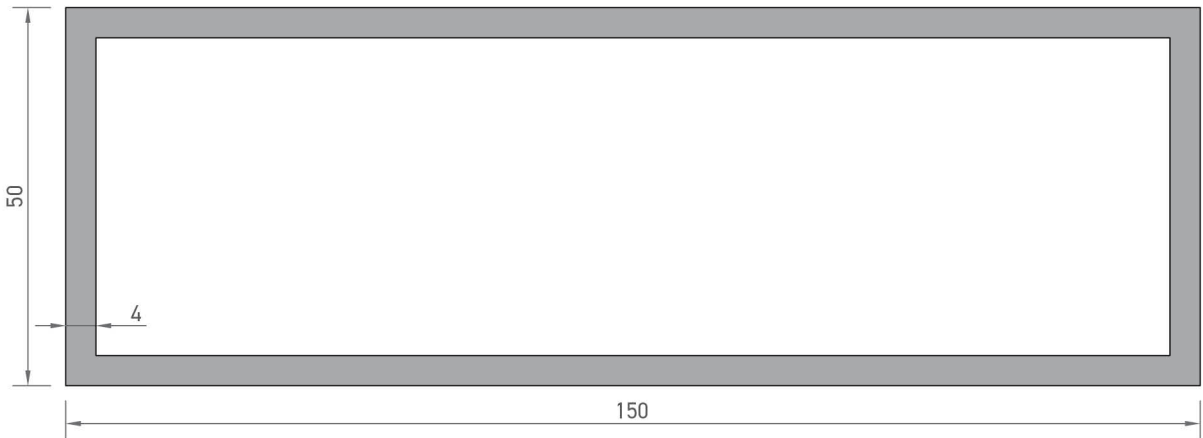
8370 KUTU PROFİLİ 4,163 kg/mt
