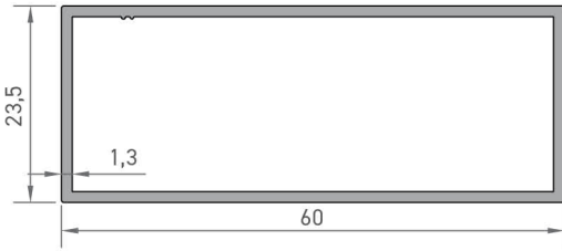
8878 KUTU PROFİLİ 0,570 kg/mt
