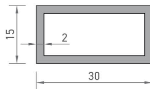
7048 KUTU PROFİLİ 0,445 kg/mt
