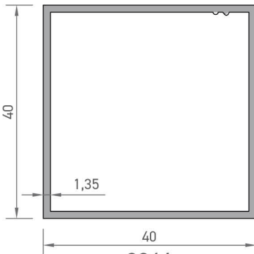
3346 KUTU PROFİLİ 0,568 kg/mt
