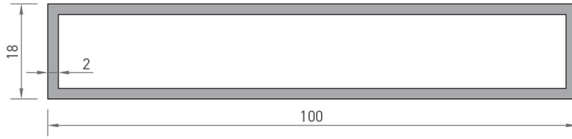
8451 KUTU PROFİLİ 1,236 kg/mt
