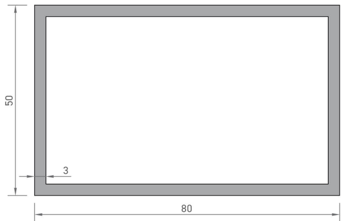
2125 KUTU PROFİLİ 2,017 kg/mt
