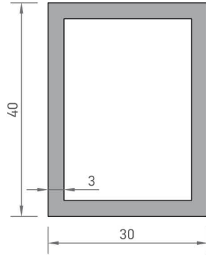
8450 KUTU PROFİLİ 1,041 kg/mt
