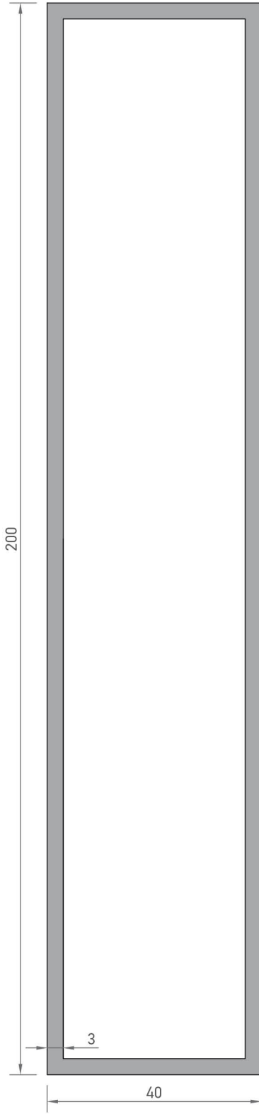
8474 KUTU PROFİLİ 3,805 kg/mt
