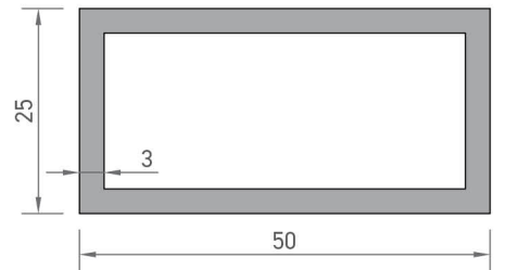
8457 KUTU PROFİLİ 1,122 kg/mt
