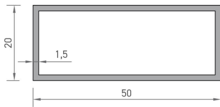
4717 KUTU PROFİLİ 0,549 kg/mt
