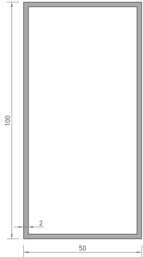
7498 KUTU PROFİLİ 1,577 kg/mt
