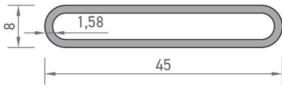
3052 KUTU PROFİLİ 0,384 kg/mt
