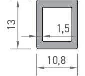
4244 KUTU PROFİLİ 0,190 kg/mt
