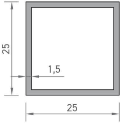
8518 KUTU PROFİLİ 0,382 kg/mt
