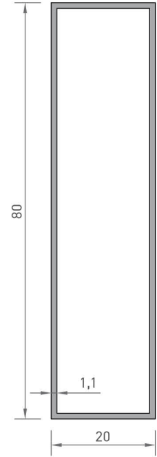
3826 KUTU PROFİLİ 0,583 kg/mt
