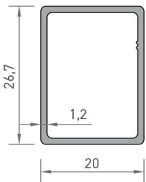
8533 KUTU PROFİLİ 0,290 kg/mt
