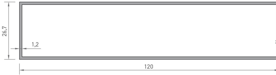
7862 KUTU PROFİLİ 0,939 kg/mt
