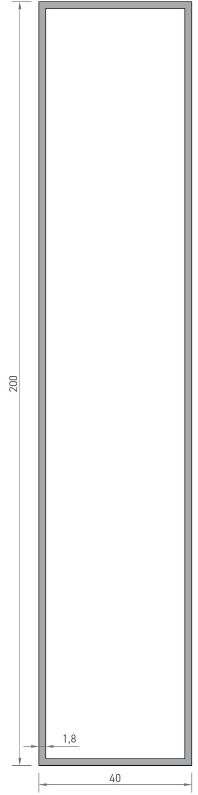
7571 KUTU PROFİLİ 2,298 kg/mt
