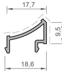
Köşe Dönüş Çıta Profili Corner Return Bead Profile
