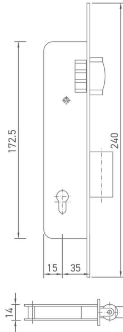
Geniş Kilit (Makaralı) Wide Type Lock (Roller) W55.782-1
