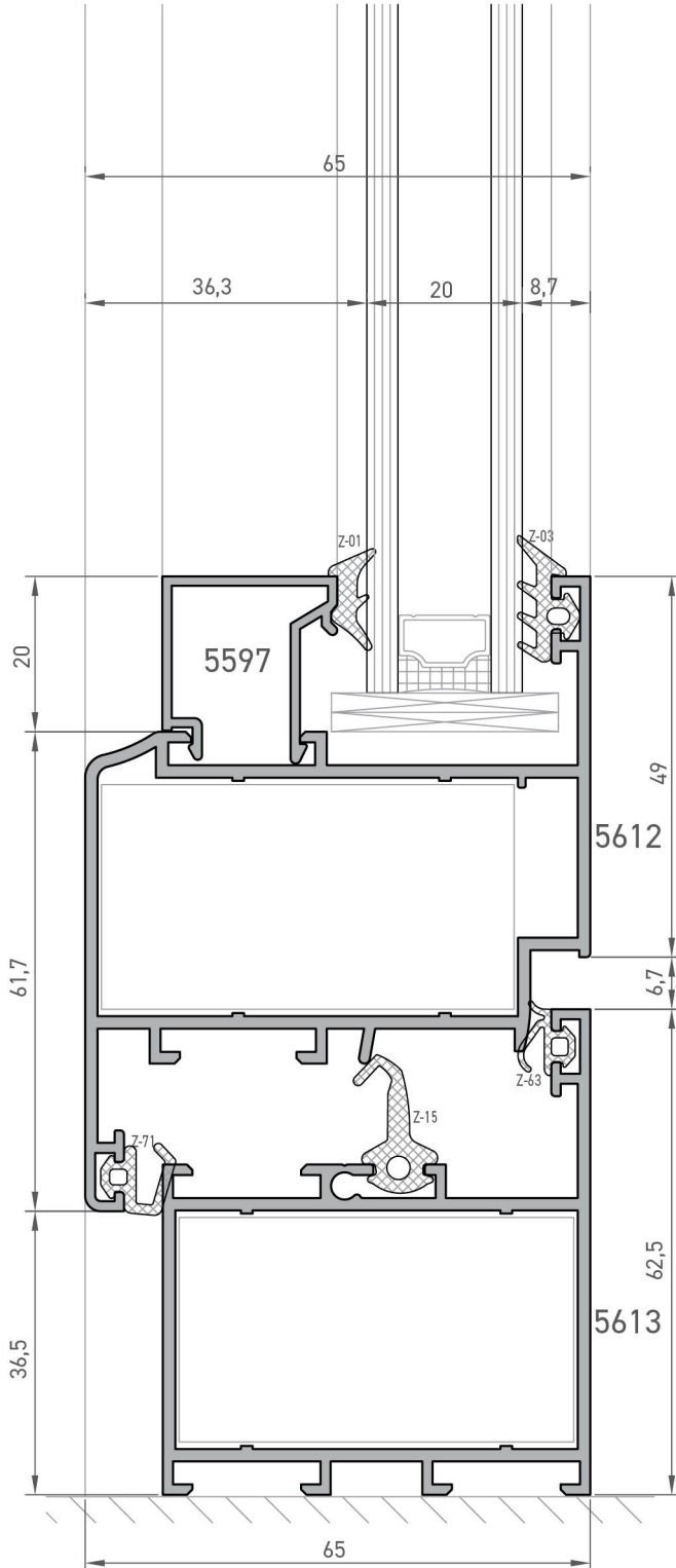
İçe Açılır Pencere Inward Opening Window
