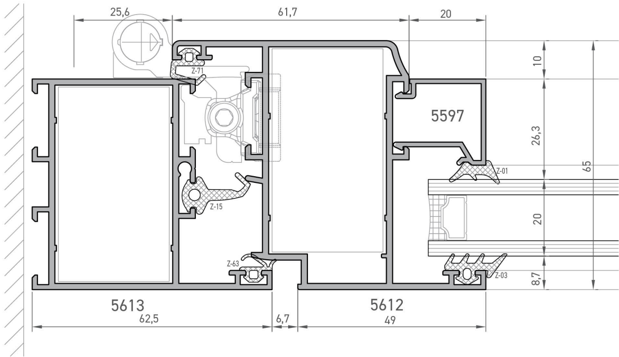
Euro Kanallı Kesit 1 euro groove section 1
