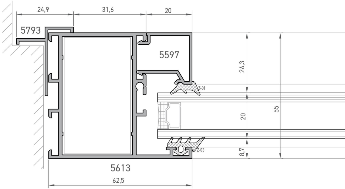
Euro Kanallı Kesit 1 euro groove section 1
