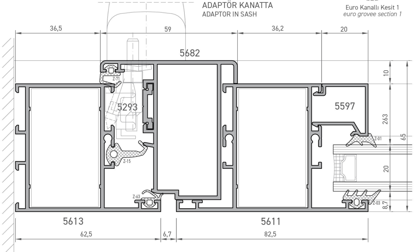
Pivot Açılır Pencere Pivot Opening Window
