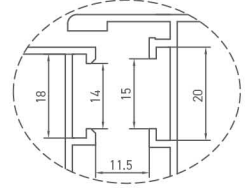
Euro Kanallı Kesit 1 euro groove section 1
