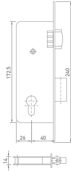
Geniş Kilit (Makaralı) Wide Type Lock (Roller) W55.782
