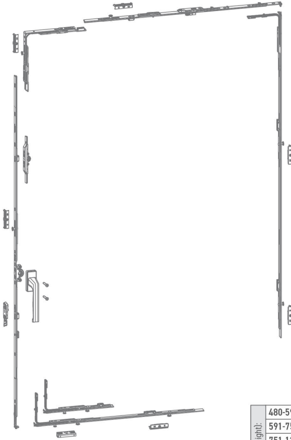
İçe Açılır Pencere Inward Opening Window
