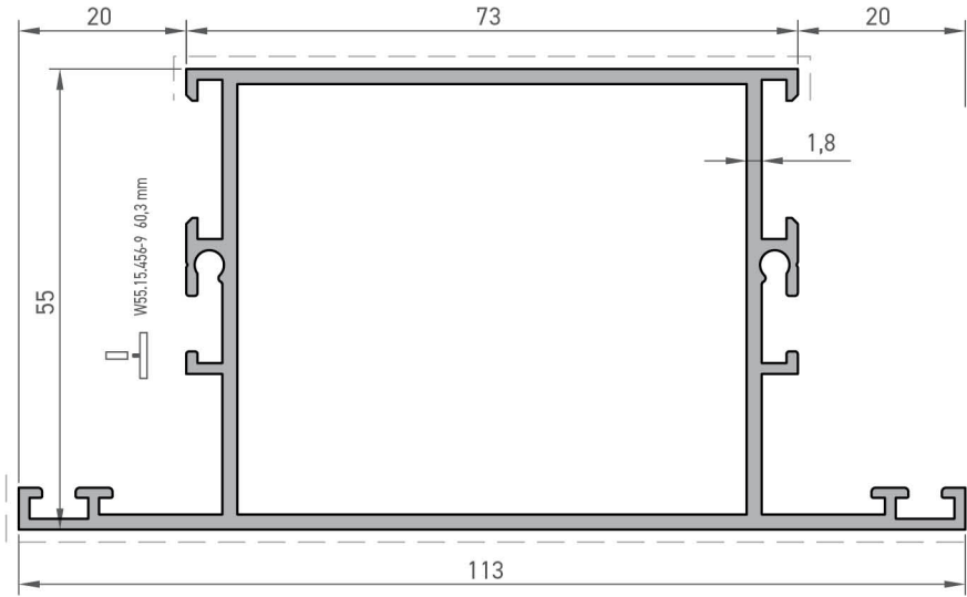
Baza Orta Kayıt Profili Base Mullion Profile
