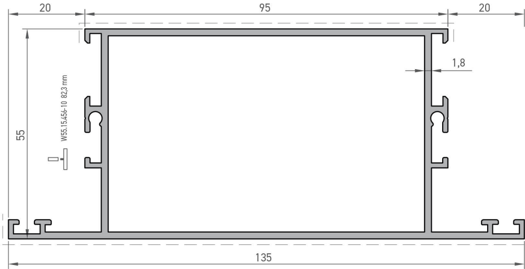
Baza Orta Kayıt Profili Base Mullion Profile
