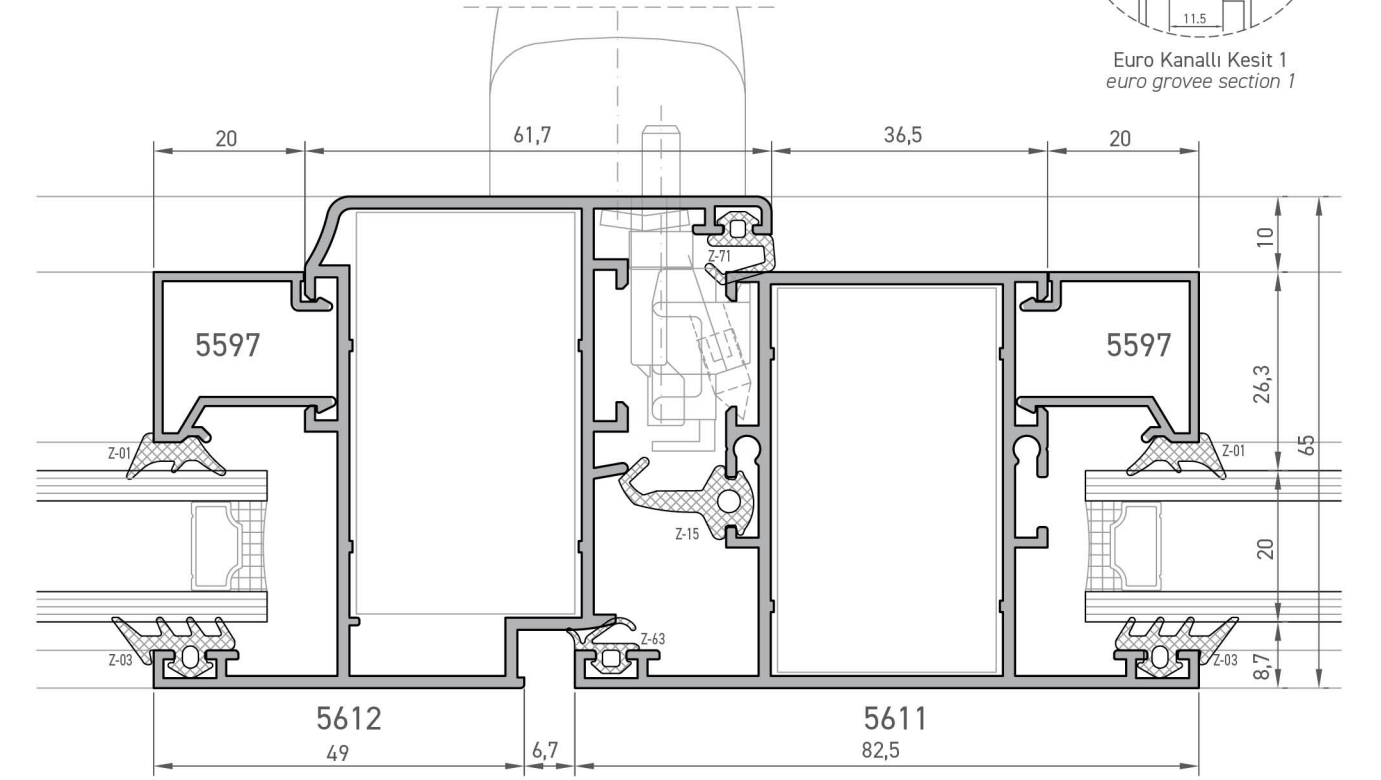
İçe Açılır Pencere Inward Opening Window
