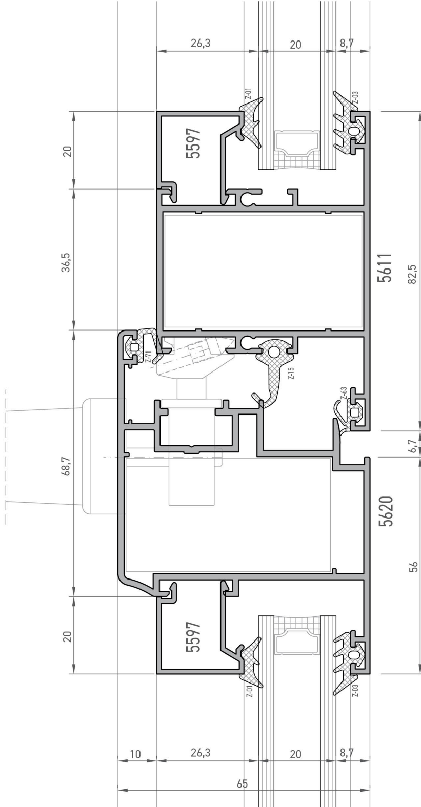
İçe Açılır Pencere Inward Opening Window
