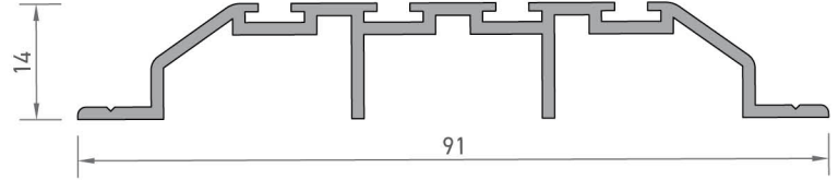
2070 SÜRME TOZLUK PROFİLİ 0,623 kg/mt
