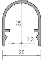
2122 20'LİK GRİYAJ ALTI PROFİLİ 0,227 kg/mt
