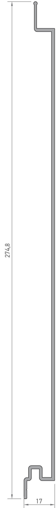
8060 YAPRAK LAMBİRİ PROFİLİ 1,483 kg/mt
