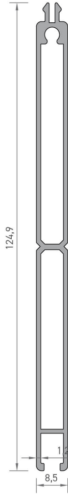
3936 LAMBİRİ PROFİLİ 0,920 kg/mt
