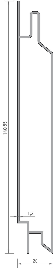
7810 LAMBİRİ PROFİLİ 1,065 kg/mt
