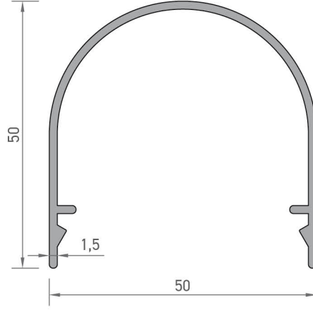
2126 20'LİK GRİYAJ ALTI PROFİLİ 0,559 kg/mt
