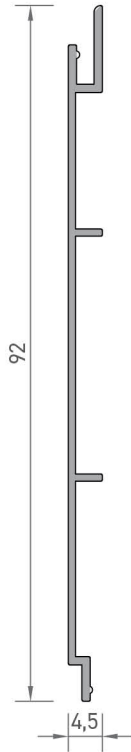
2114 LAMBİRİ PROFİLİ 0,296 kg/mt
