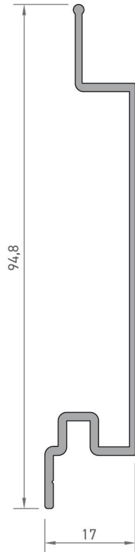
6005 LAMBİRİ PROFİLİ 0,467 kg/mt
