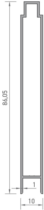
2115 TAHTA LAMBİRİ PROFİLİ 0,509 kg/mt
