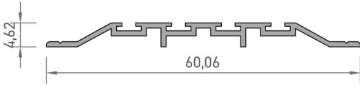
2045 SÜRME TOZLUK PROFİLİ 0,507 kg/mt
