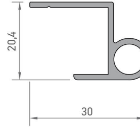
6708 BAĞLANTI PROFİLİ 0,270 kg/mt
