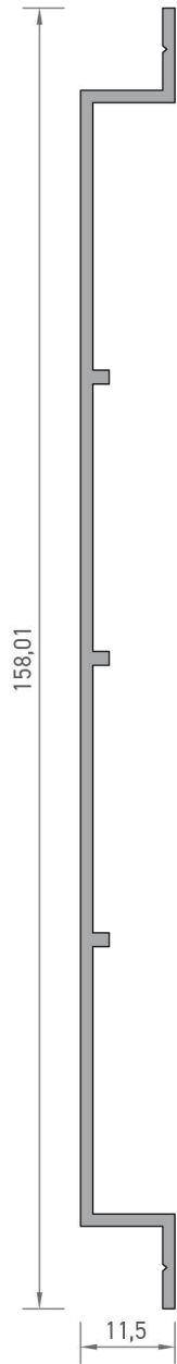
3953 LAMBİRİ PROFİLİ 0,750 kg/mt
