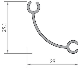
6707 BAĞLANTI PROFİLİ 0,216 kg/mt
