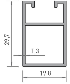
2743 REKLAM PROFİLİ 0,372 kg/mt
