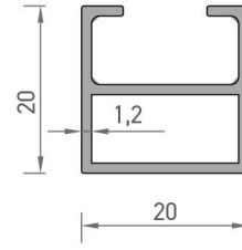
3158 REKLAM PROFİLİ 0,275 kg/mt
