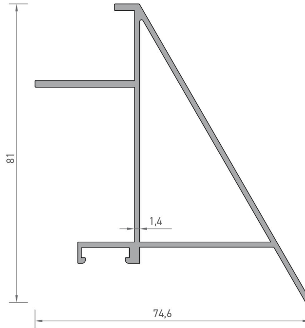
1968 YAN ÇERÇEVE PROFİLİ 1,010 kg/mt
