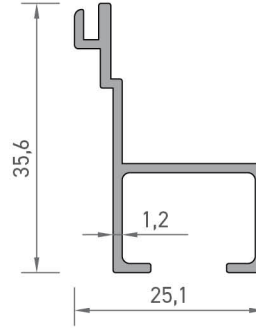
3159 REKLAM PROFİLİ 0,285 kg/mt
