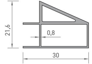
2965 YAN ÇERÇEVE PROFİLİ 4,275 kg/mt
