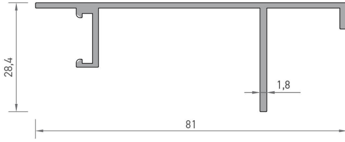
1967 REKLAM PROFİLİ 0,565 kg/mt
